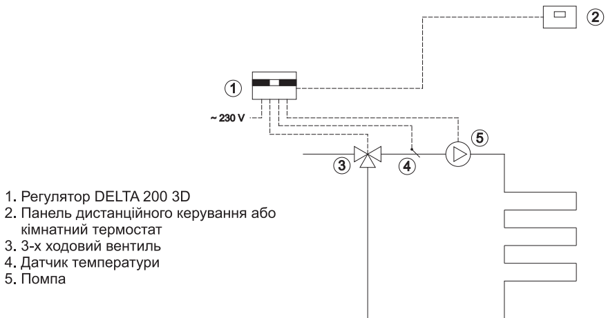
Рис. 1 Підключення регулятора до інсталяції підлогового опалення
