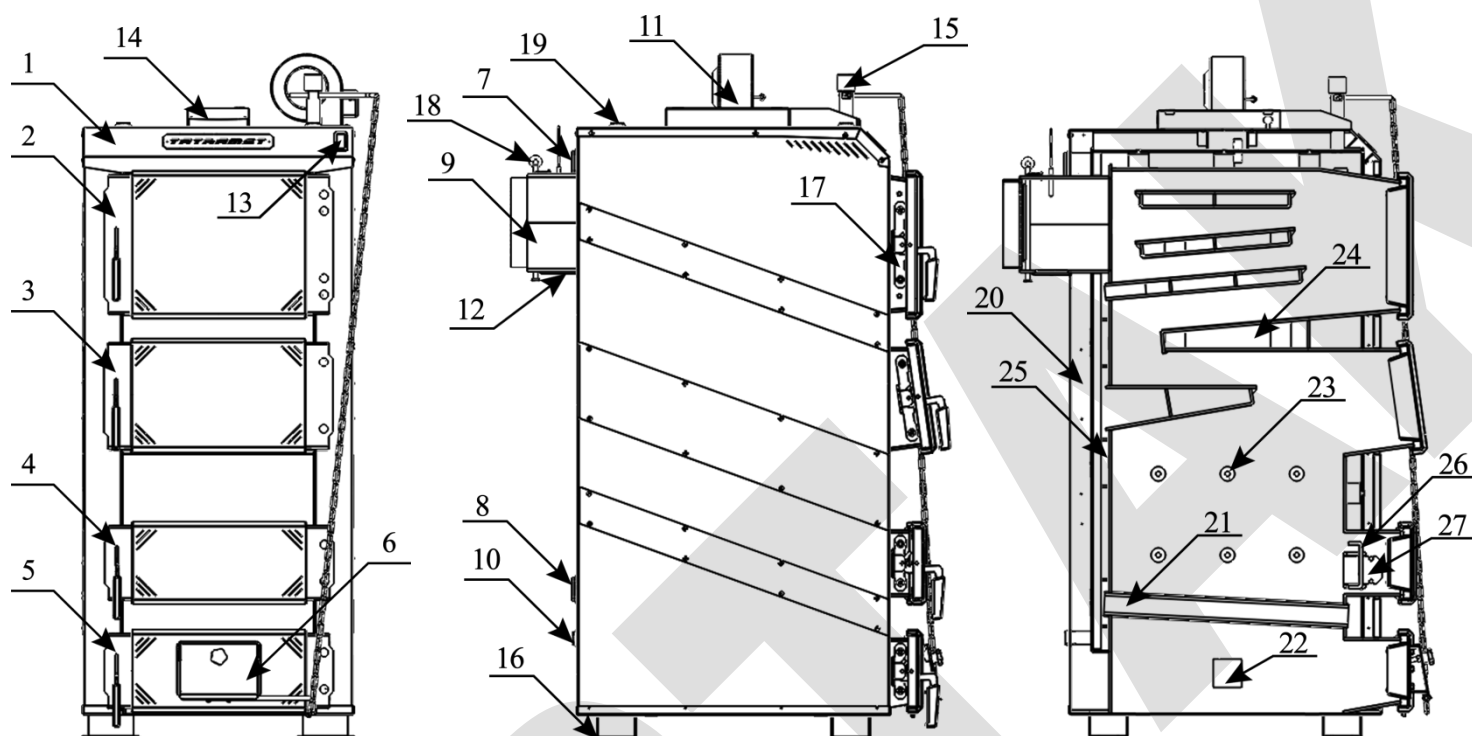
Рис. 3 Специфікація елементів котлів типу SPARTAK Plus
