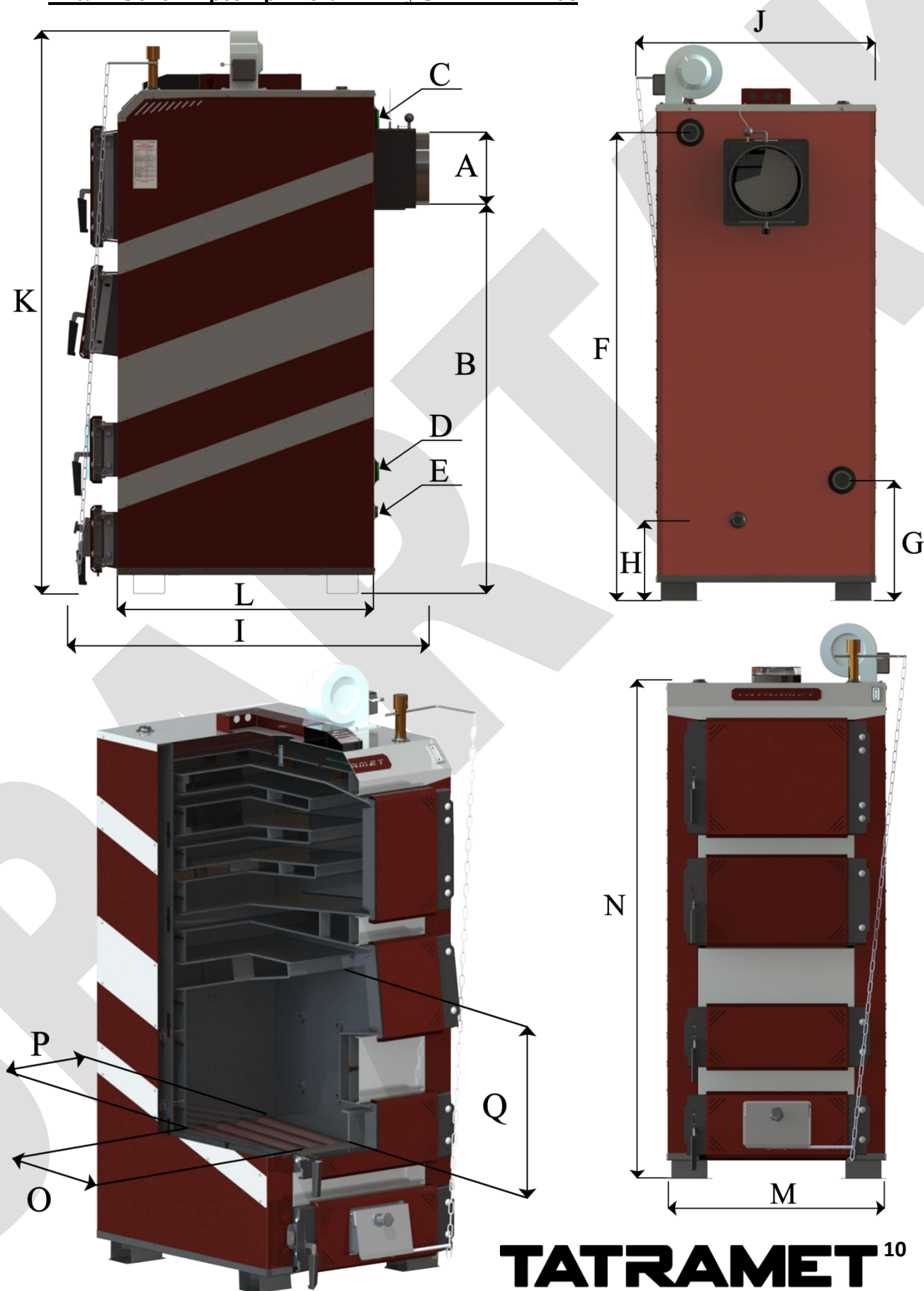
Рис. 2 Основні розміри котлів типу SPARTAK Plus
