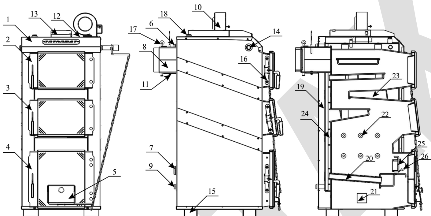
Рис. 3 Специфікація елементів котлів типу SPARTAK Uni
