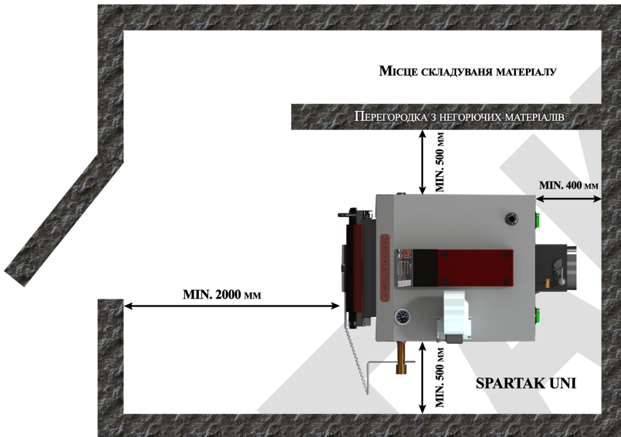
Рис.4 Схема монтажу котла в приміщенні котельної
