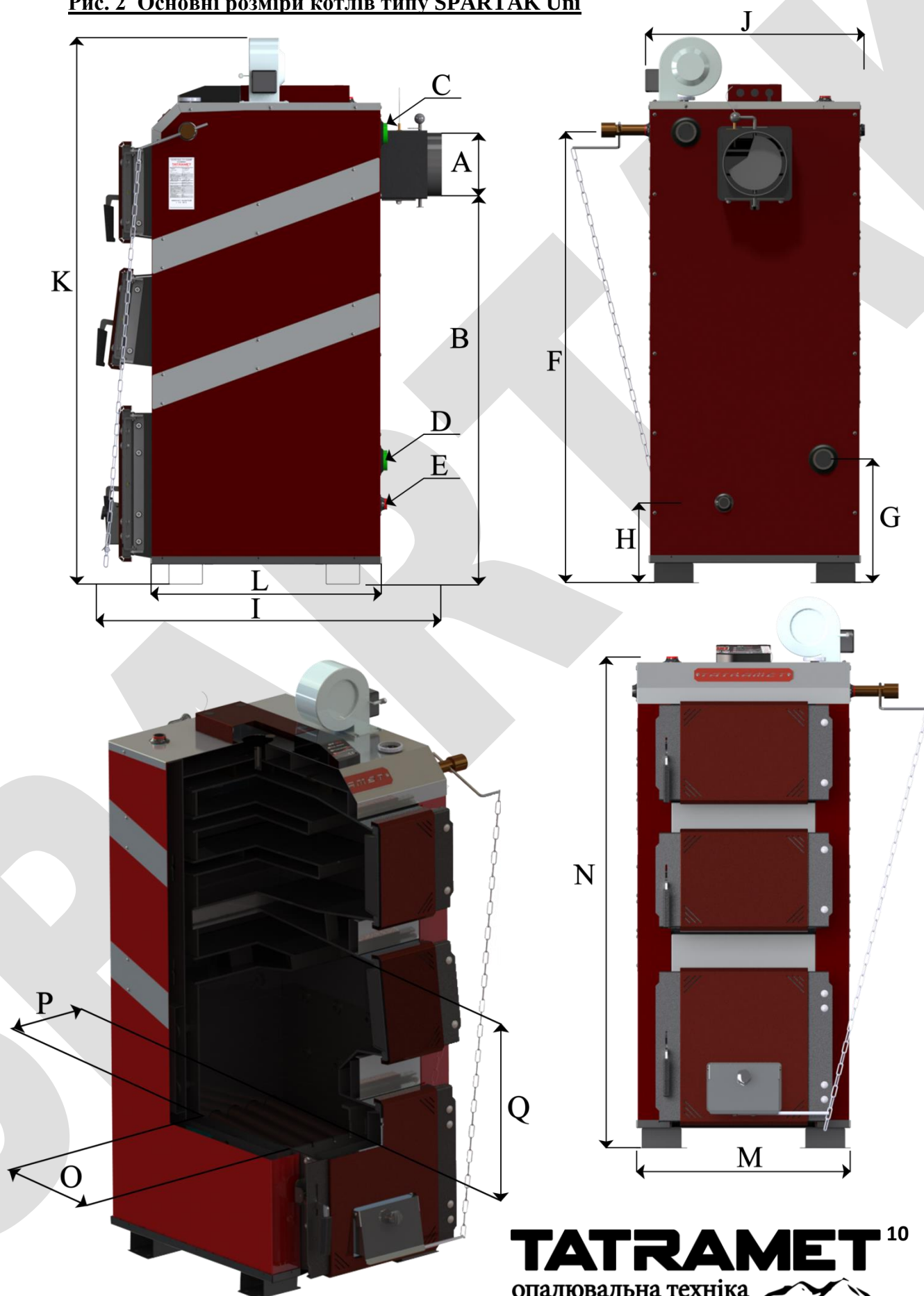
Рис. 2 Основні розміри котлів типу SPARTAK Uni
