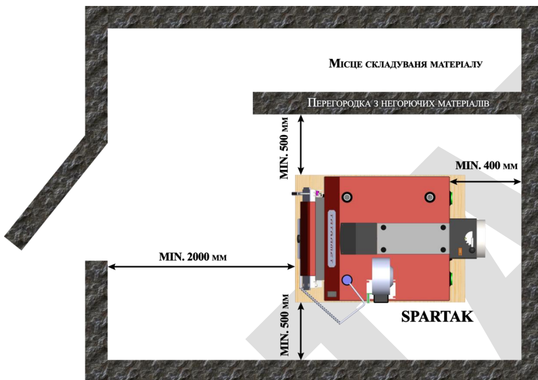
Рис.4 Схема монтажу котла в приміщенні котельної
