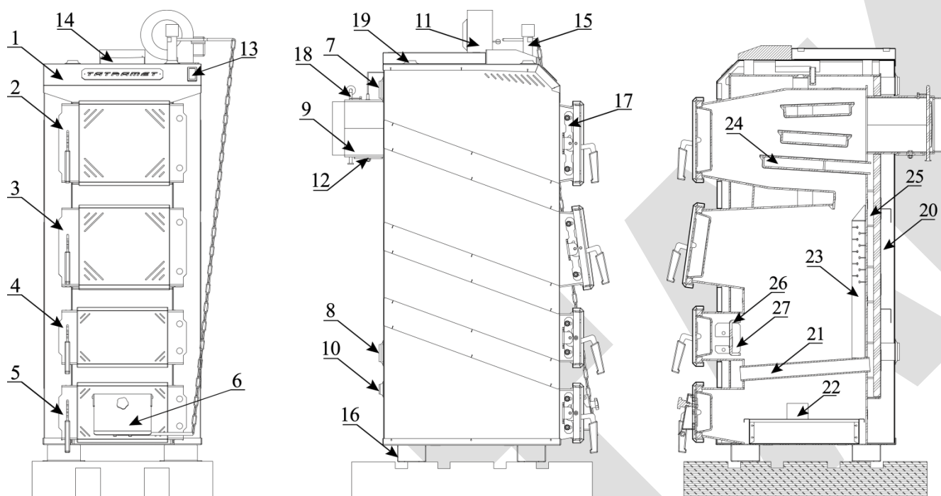
Рис. 3 Специфікація елементів котлів типу SPARTAK
