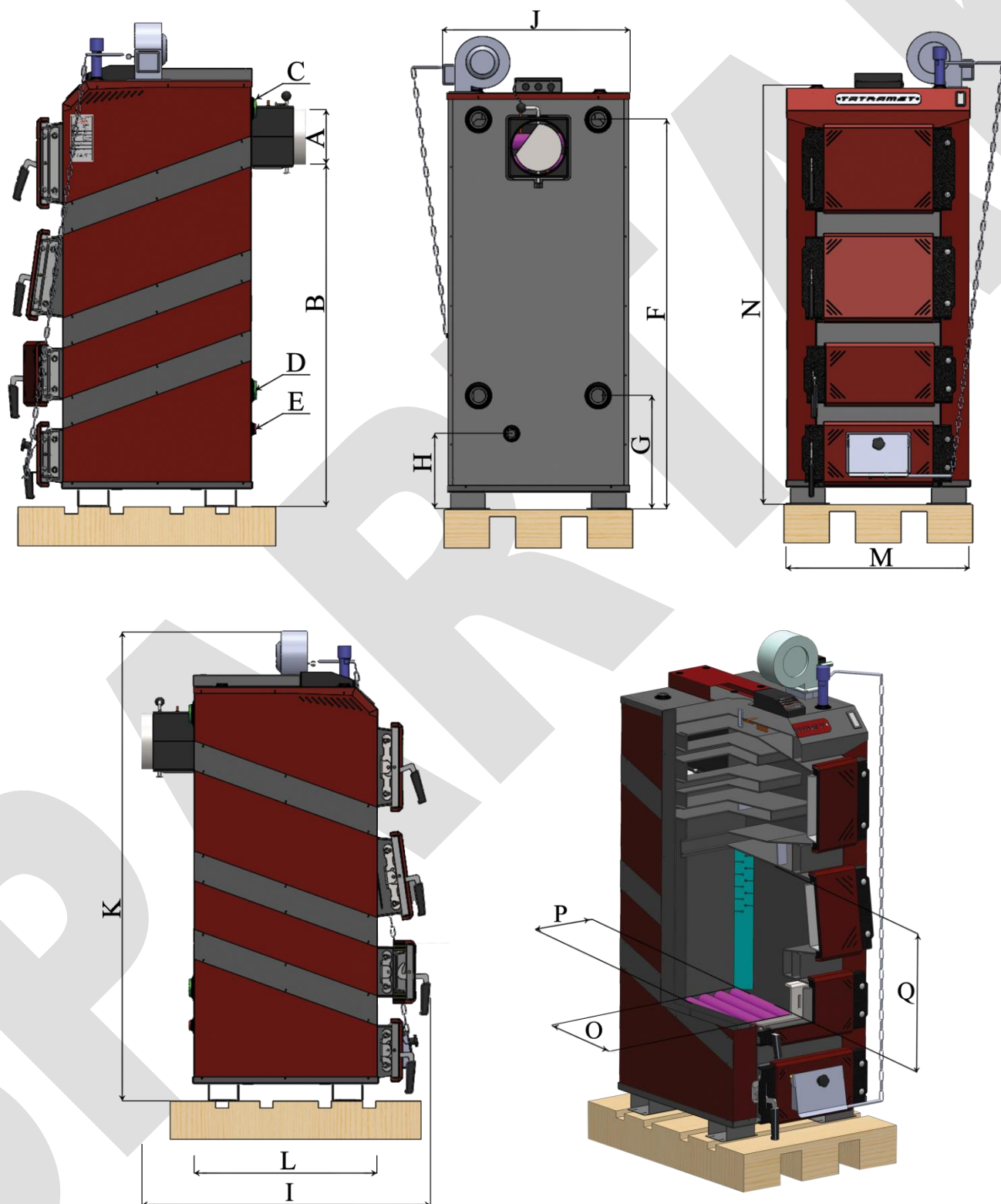
Рис. 2 Основні розміри котлів типу SPARTAK
