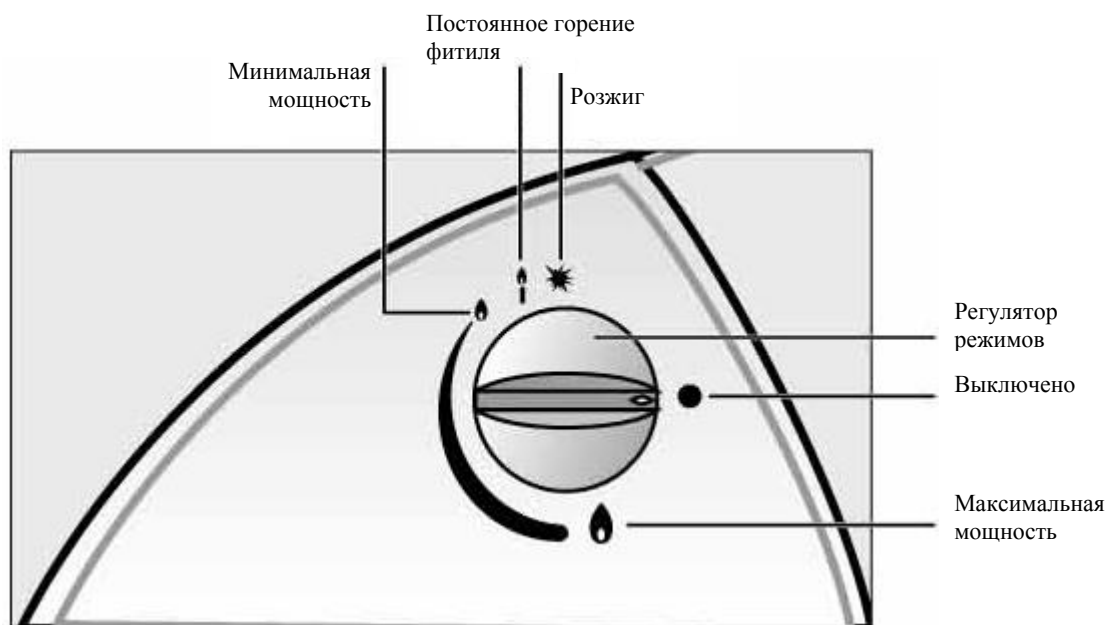
Рисунок 2. Панель управления водонагревателей серии B.
